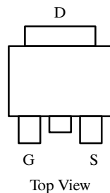
DPAK (TO-252)
